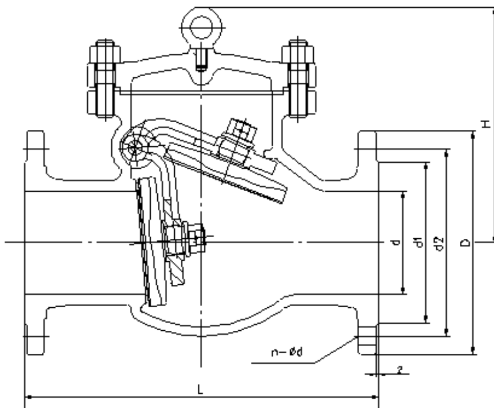
PN25 DIN Check Valve
