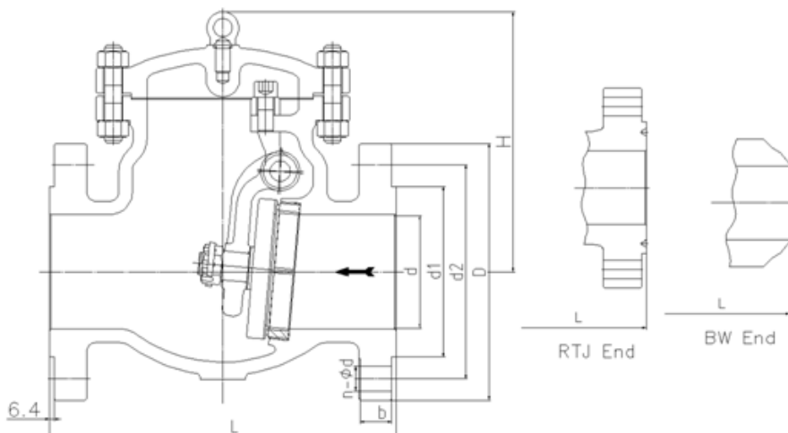
Class900 Non Return Valve
