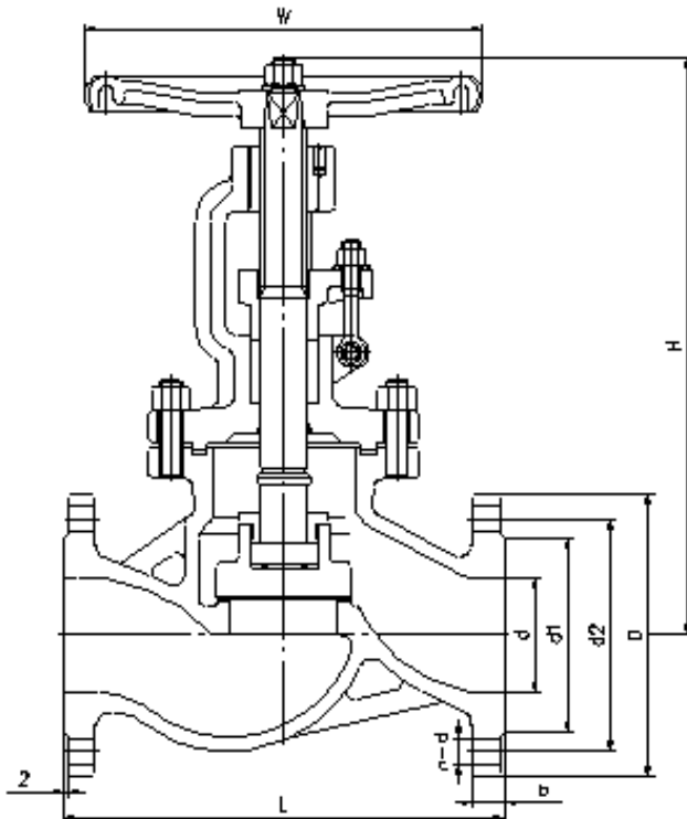
PN40 DIN3356 Golbe Valve
